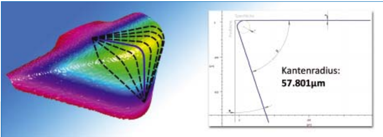
Der Kantenradius bzw. die Verrundung, hier gemessen mit dem Alicona Schneidkantenmessgerät IF-EdgeMaster, entscheiden über Kantestärke und Oberflächenqualität des bearbeiteten Werkstücks.
