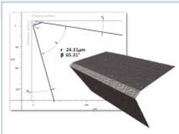
Optimierte Fasengeometrien, hier Messung einer Negativfase, können Verschleiß verringern und damit die Standzeiten erhöhen.
